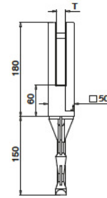
Scellement béton
